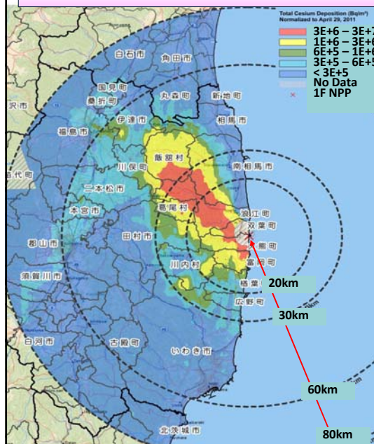
Fig. Results of total deposition of Cs-134 and Cs-137
